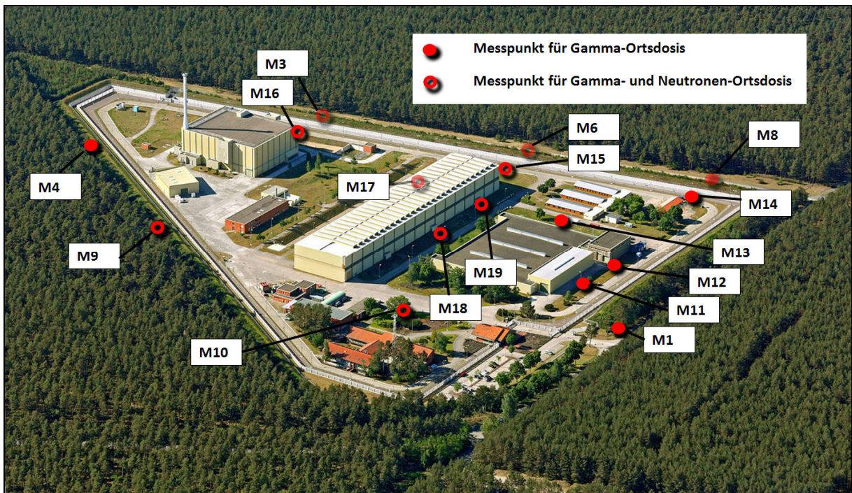
Abbildung 2: OD-Messpunkte
